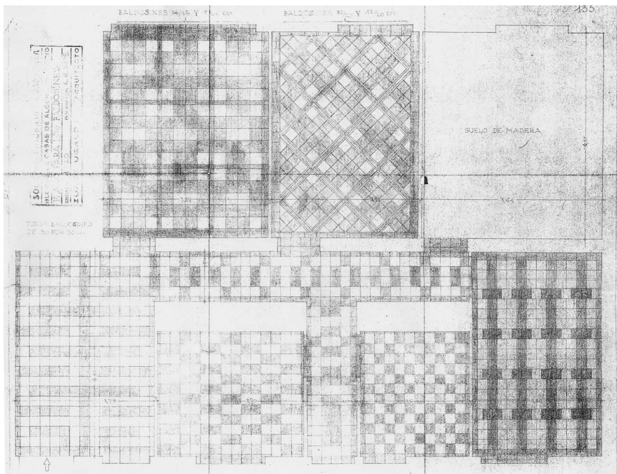
Plano de solado en una vivienda firmado por Zuazo en marzo de 1931. Reproducción del Servicio Histórico del COAM.
