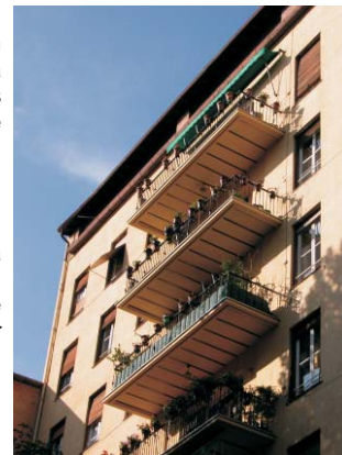
Arriba: Hilarion Eslava 2 hacia jardín Abajo: Detalle inferior de las bandejas con el paño central rehundido y su borde regresado. Fotografías: MMN Arquitectos. Oct. 2003.
